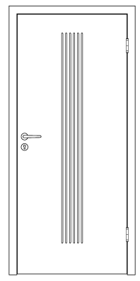
Typ Lombardo 2800-7 Zierfräsungen aufrecht
