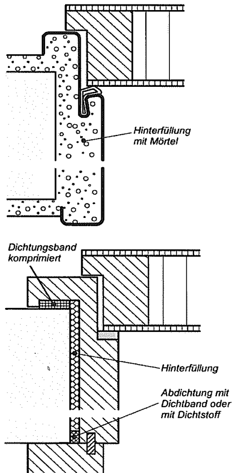
Bild 11 Hinterfüllungs- und Abdichtungsmaßnahmen an Türzarge
