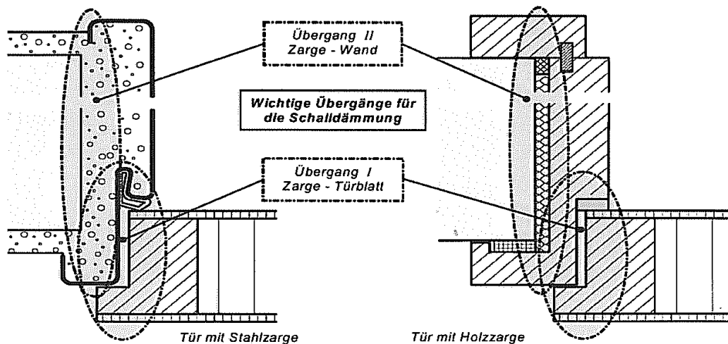
Bild 7 Wichtige Abdichtungsbereiche bei Türen
