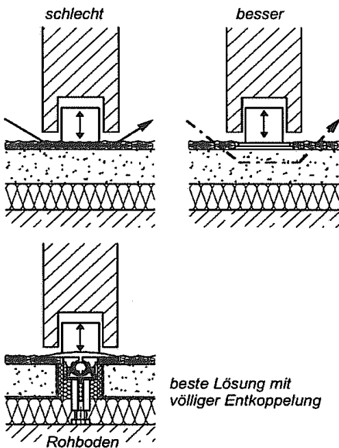
Bild 10 Schallübertragungswege u. Entkoppelungsmaßnahmen im Fußbodenanschlussbereich
