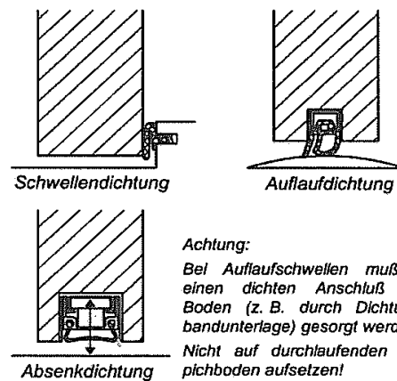
Bild 9 Abdichtungsmöglichkeiten zwischen Tür und Fußboden
