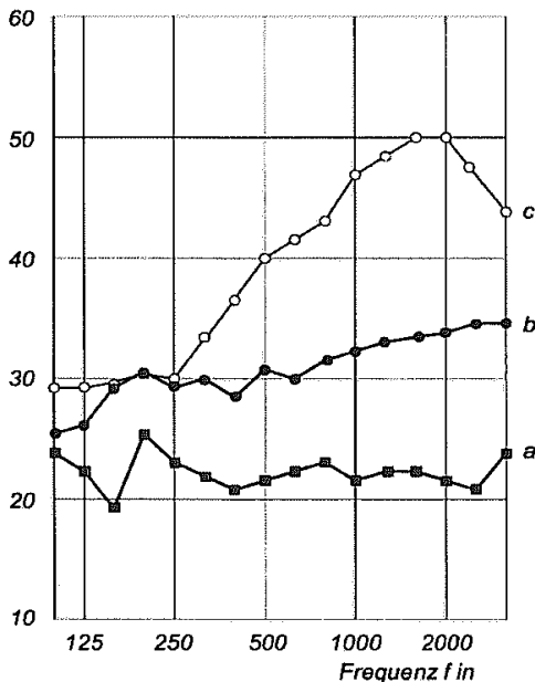
Schalldämm-Maß in dB
