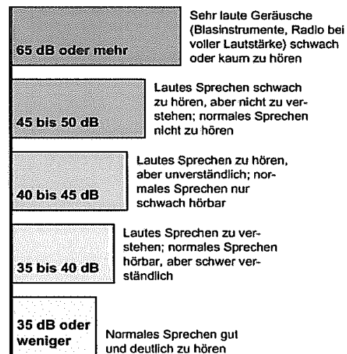
Bild 2 Bewertetes Schalldämmmaß – Höreindruck nach der Schalldämmung
