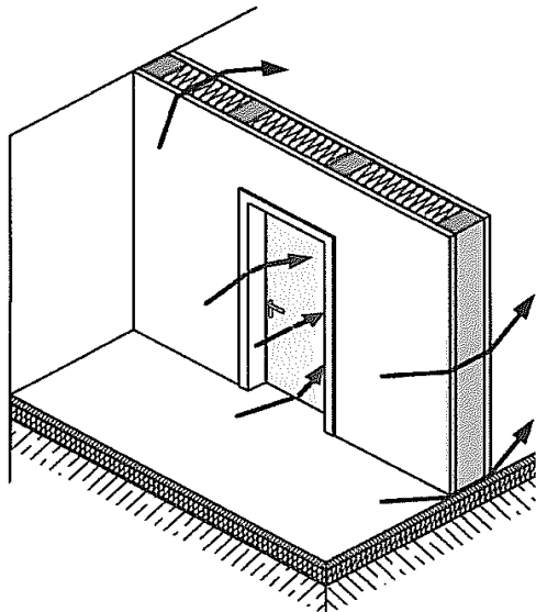
Bild 3 Schallübertragungswege bei einer Trennwand mit Verbindungstür
